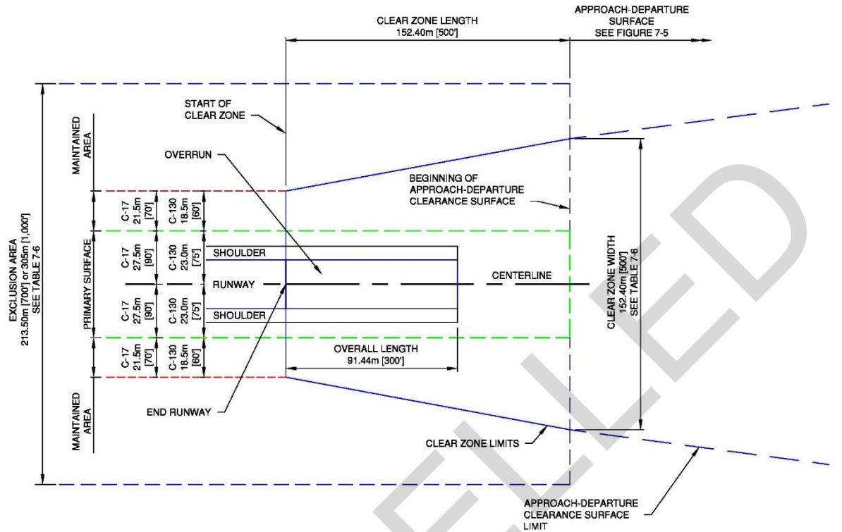
PLAN N.T.S.
