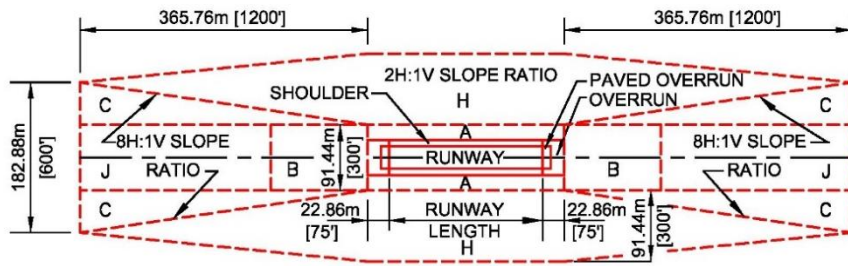
PLAN N.T.S.
