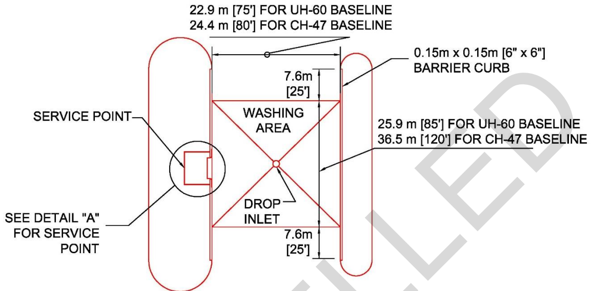
PLAN N.T.S.
