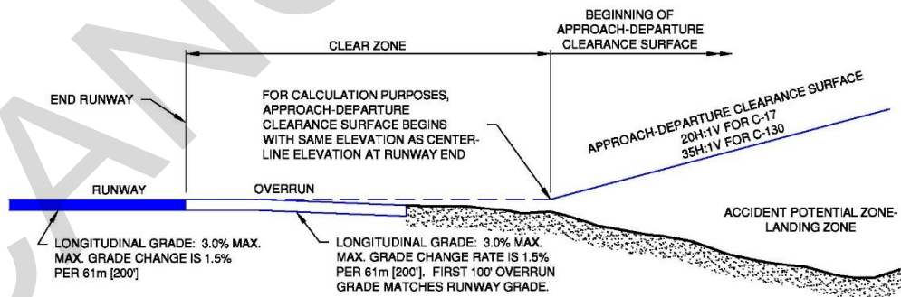
LONGITUDINAL PROFILE N.T.S.
