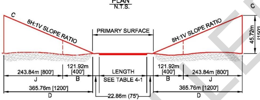
LONGITUDINAL PROFILE N.T.S.
