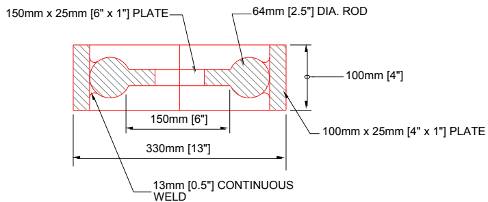
SECTION E-E N.T.S.
