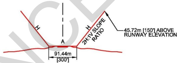
TRANSVERSE SECTION N.T.S.
